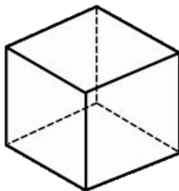
Куб {4,3}
