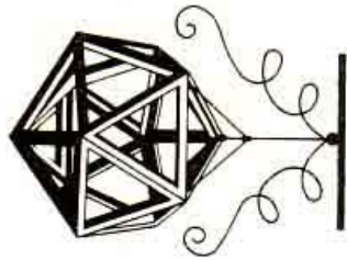
ИКОСАЭДР
