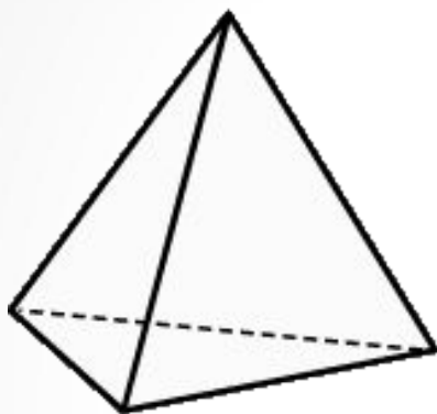
Тетраэдр {3,3}
