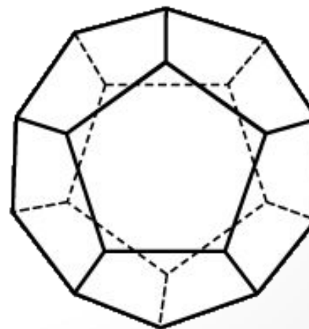
Додекаэдр {5,3}
