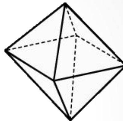
Октаэдр {3,4}
