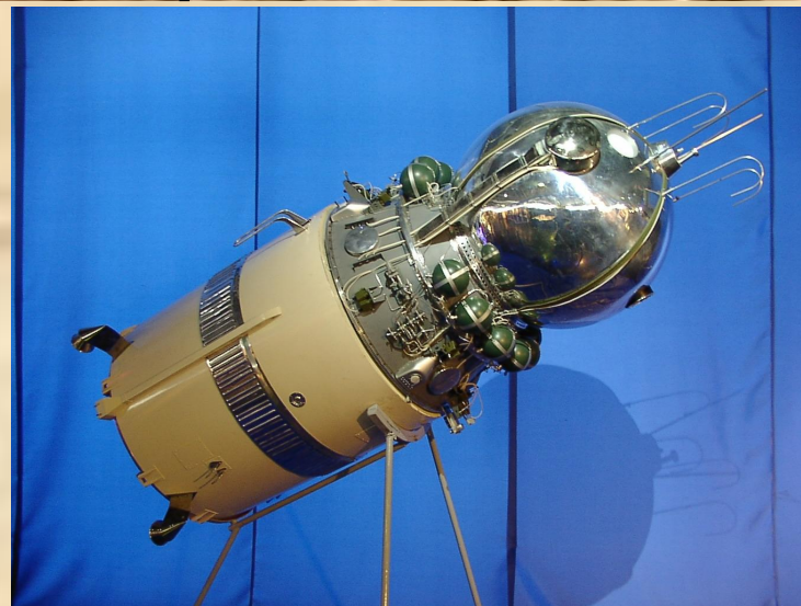
Модель космического корабля «Восток»
