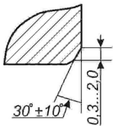
Г-Г M 1:1
