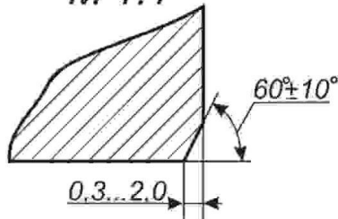
Д-Д M 1:1
