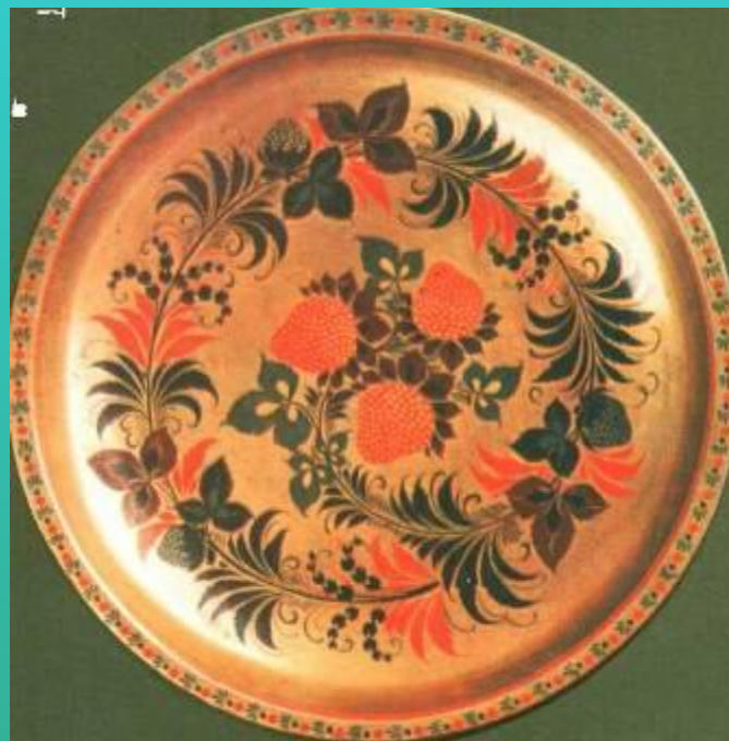
Блюдо
