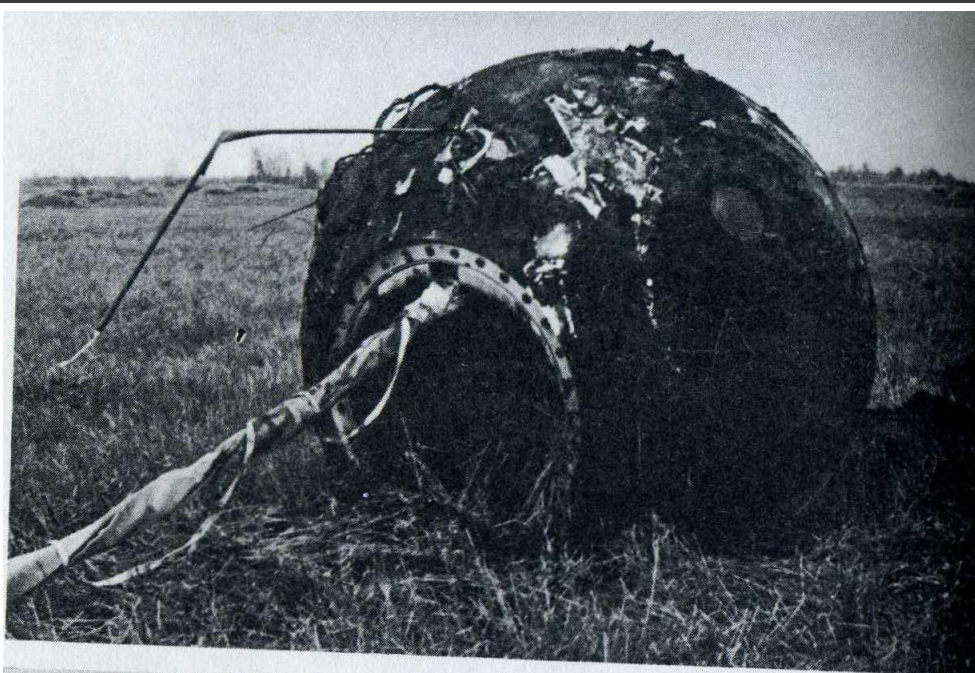
Спускаемый аппарат. В котором приземлился Юрий Гагарин.
