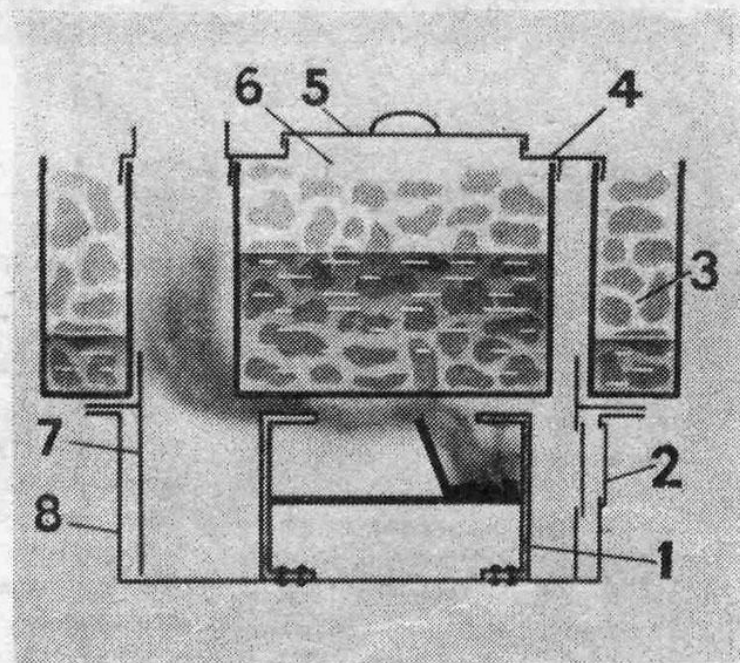
Печка для зимних туристских походов: 1 — таган для сжигания топлива; 2 — дверца топливи; 3 — бак для таяния льда; 4 — крепежная крышка; 5 — крышка; 6 — большая кастрюля; 7 — кольцо; 8 — поддон.
