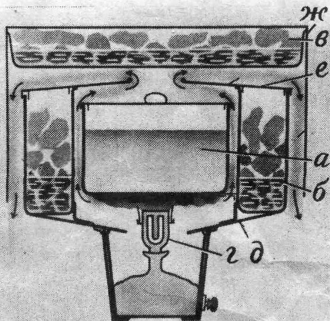
Кухонный аппарат Фритъофа Нансена: а — сосуд для варки пищи; б — кольцообразный котел для таяния льда и снега; в — плоский котел для льда и снега; г — газокеросиновая горелка «примус»; д — подставка для кольцообразного котла; е — крышка с отверстием посредине; ж — наружный колпак.
