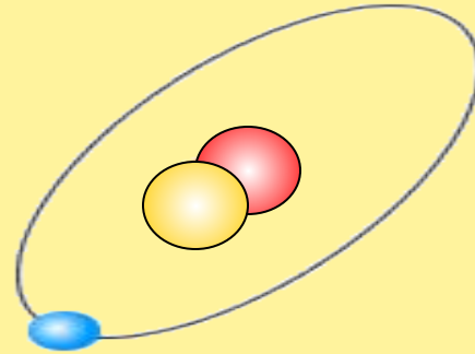
Дейтерий
