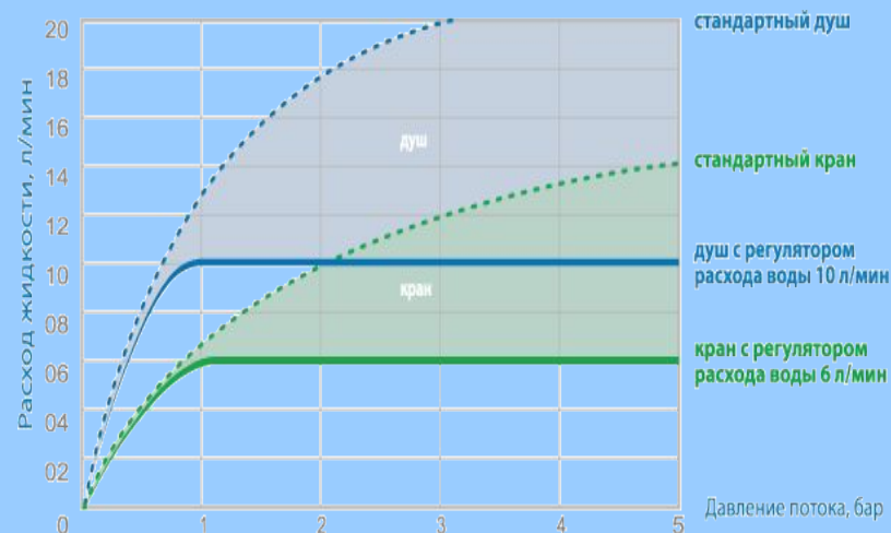
График расхода воды с РРВ и без него
