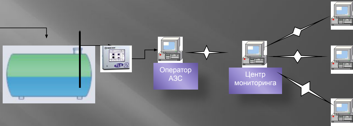
Датчик Veeder-Root
