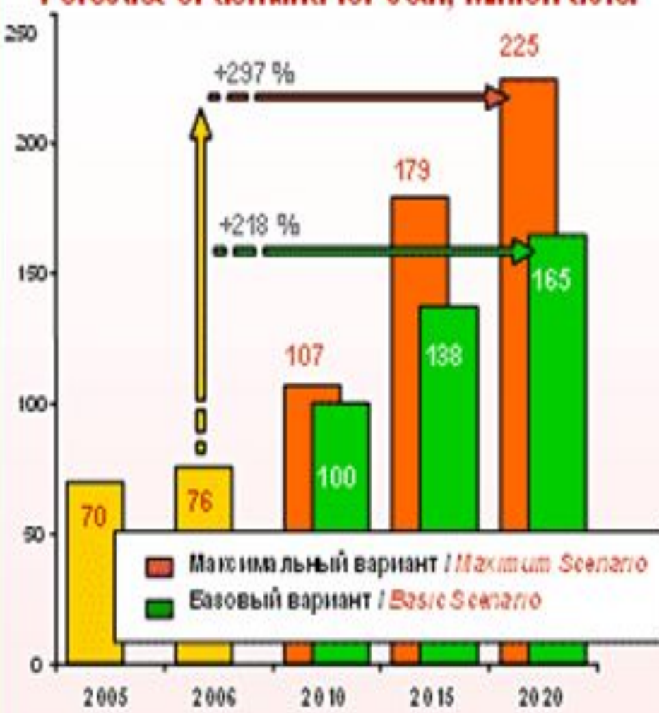
Прогноз спроса на уголь, млн т у.т. / Forecast of demand for coal, Million t.c.e.
