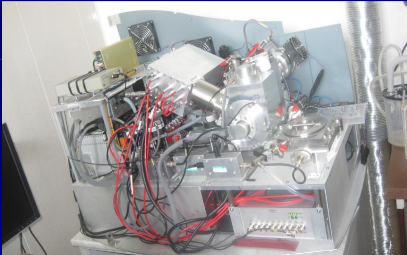
Настоящий масс-спектрограф
