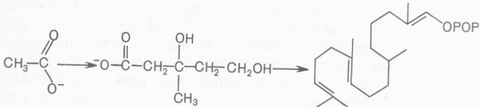
Геранил-гераниол-пирофосфат
