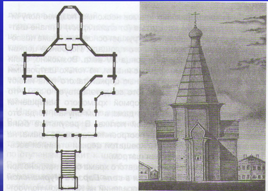
Ил. 12. План и вид Богородицкой церкви (1726 г.) в с. Заостровье Архангельской обл.
