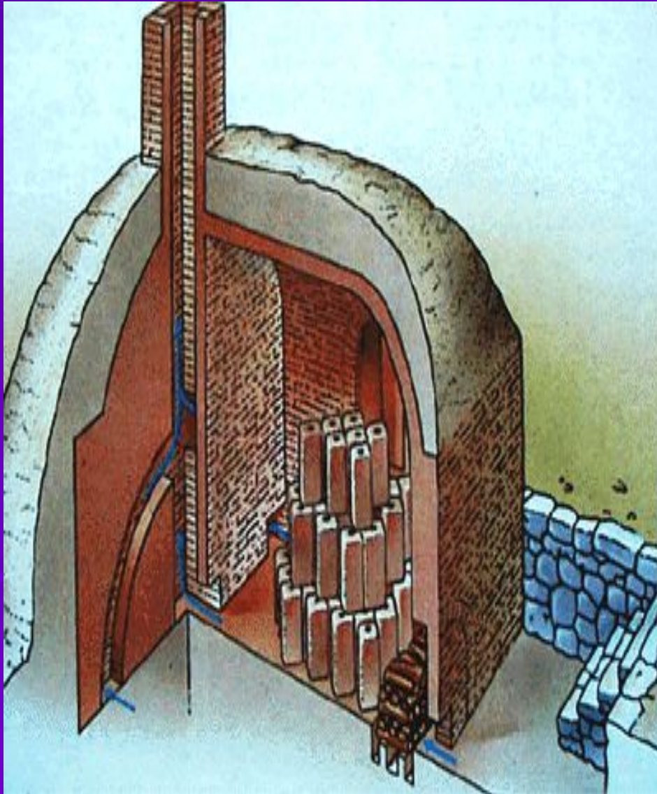
Печь для производства железа
