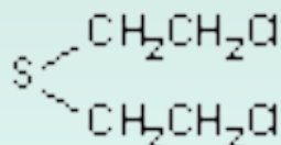
иприт
