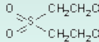
сульфон иприта
