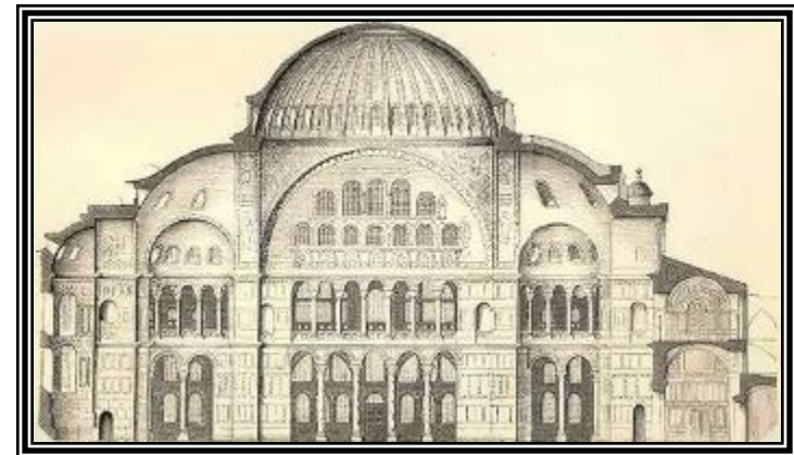
Храм Святой Софии в Константинополе. 532-537.
