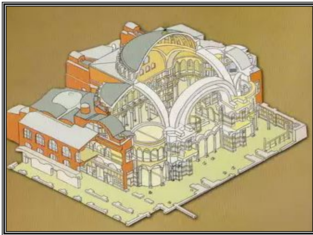
Храм Святой Софии в Константинополе. 532-537.
