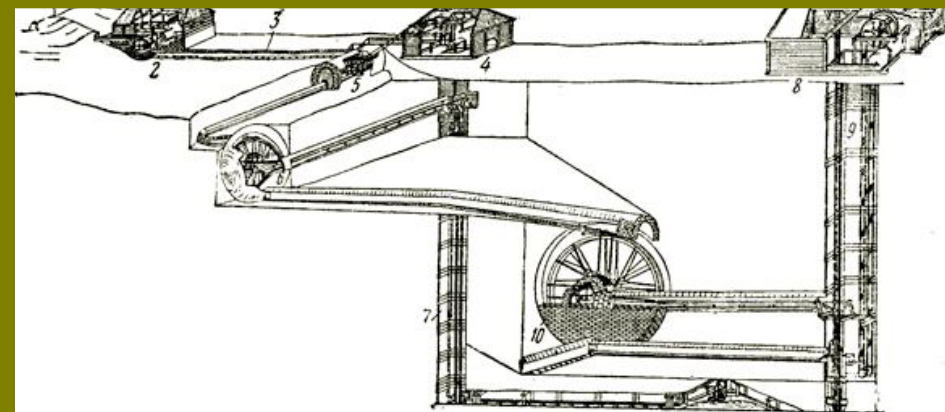
Машина для откачивания воды из шахты (Змеигородский рудник)
