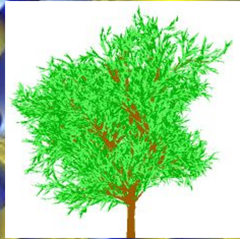
Фрактальное дерево
