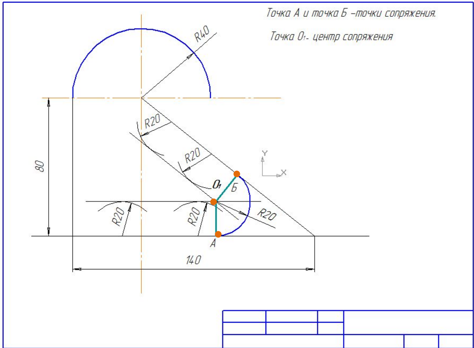
13. Наносим все точки на чертеже: точку O_1 - центр сопряжения, точку А и точку Б – точки сопряжения.
