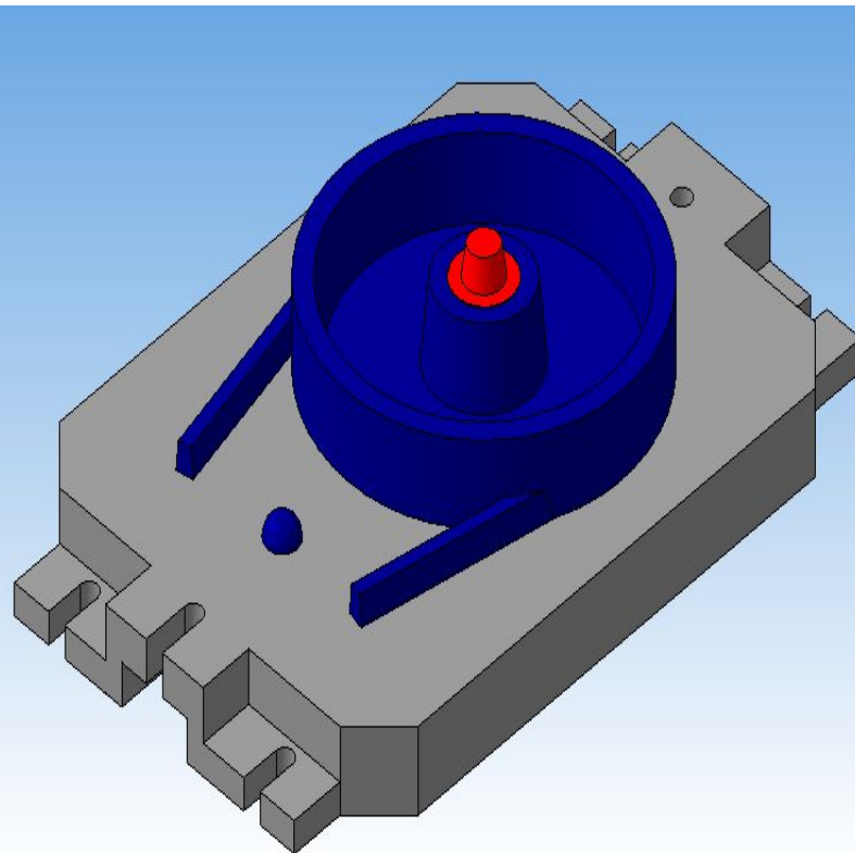
Модельная плита для изготовления нижней полуформы
