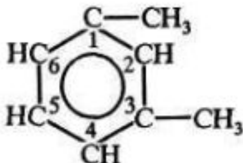
1,3-диметилбензол (м-ксилол)
