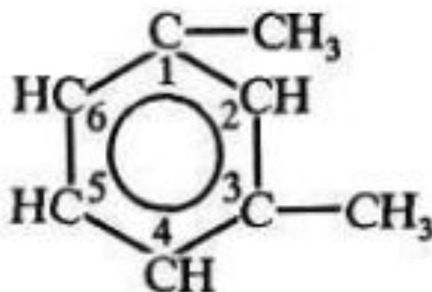
1,3-диметилбензол (м-ксилол)
