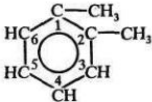
1,2-диметилбензол (о-ксилол)
