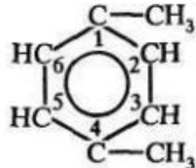
1,4-диметилбензол (п-ксилол)
