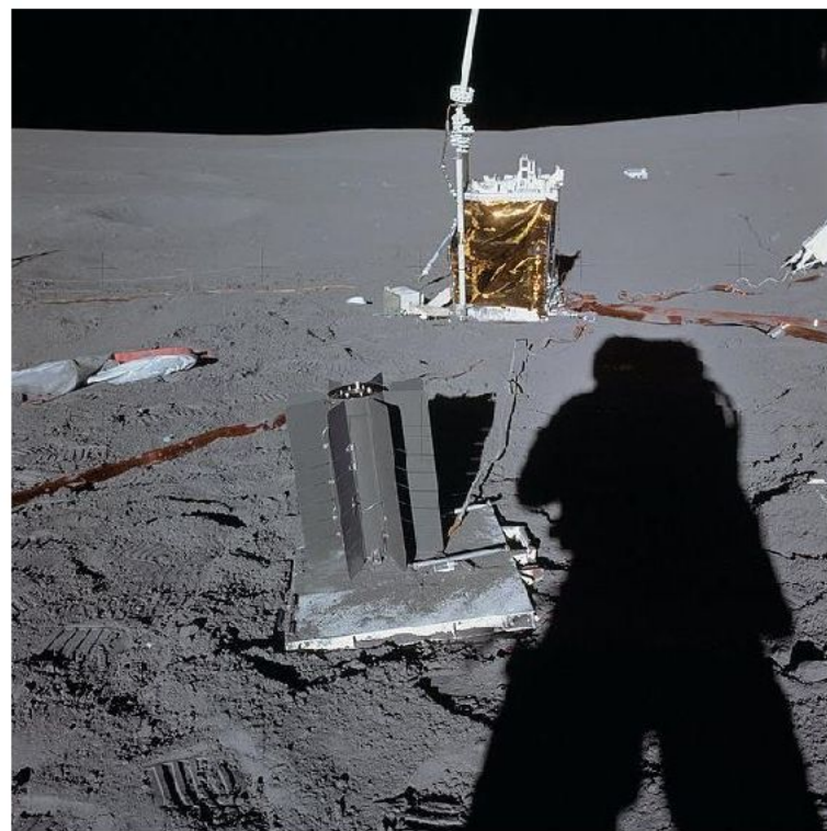
SNAP-27, Аполлон-14.
