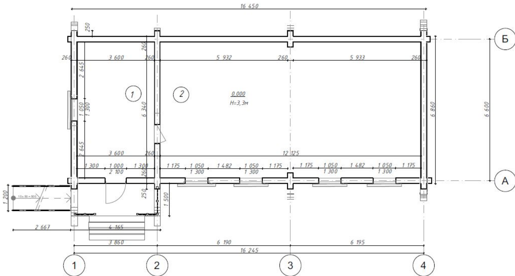
План помещений
