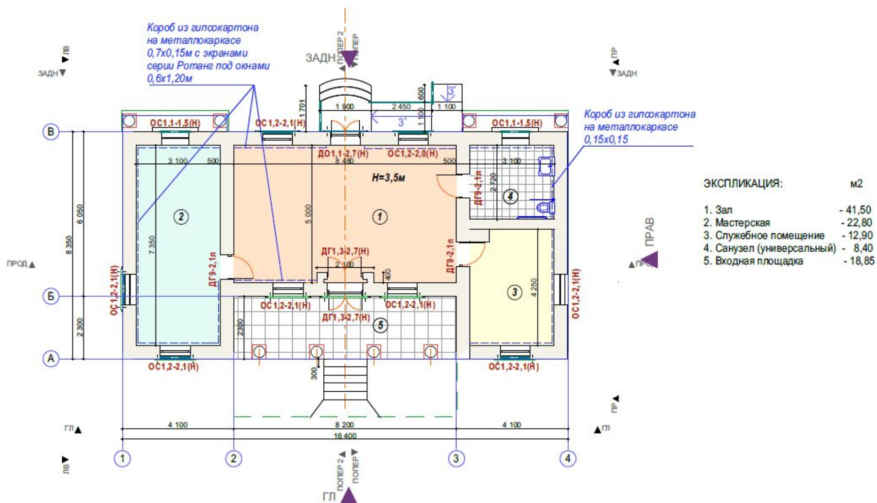
План помещений
