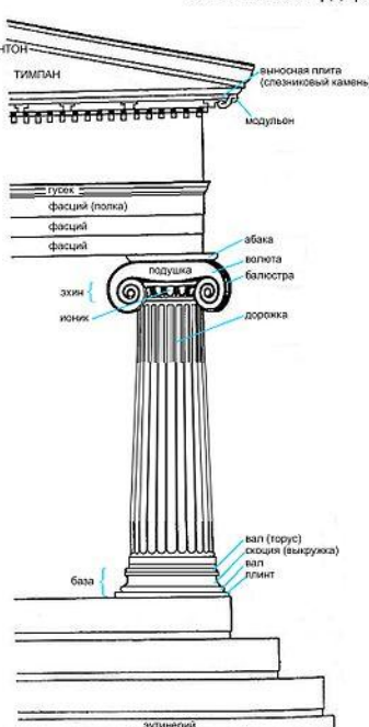
Ионический ордер
