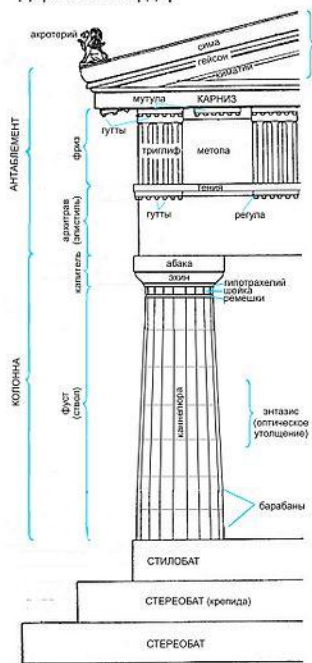
Дорический ордер
