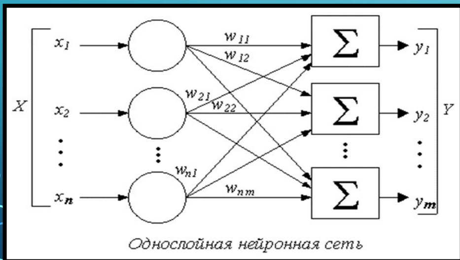
Однослойные нейронные сети
