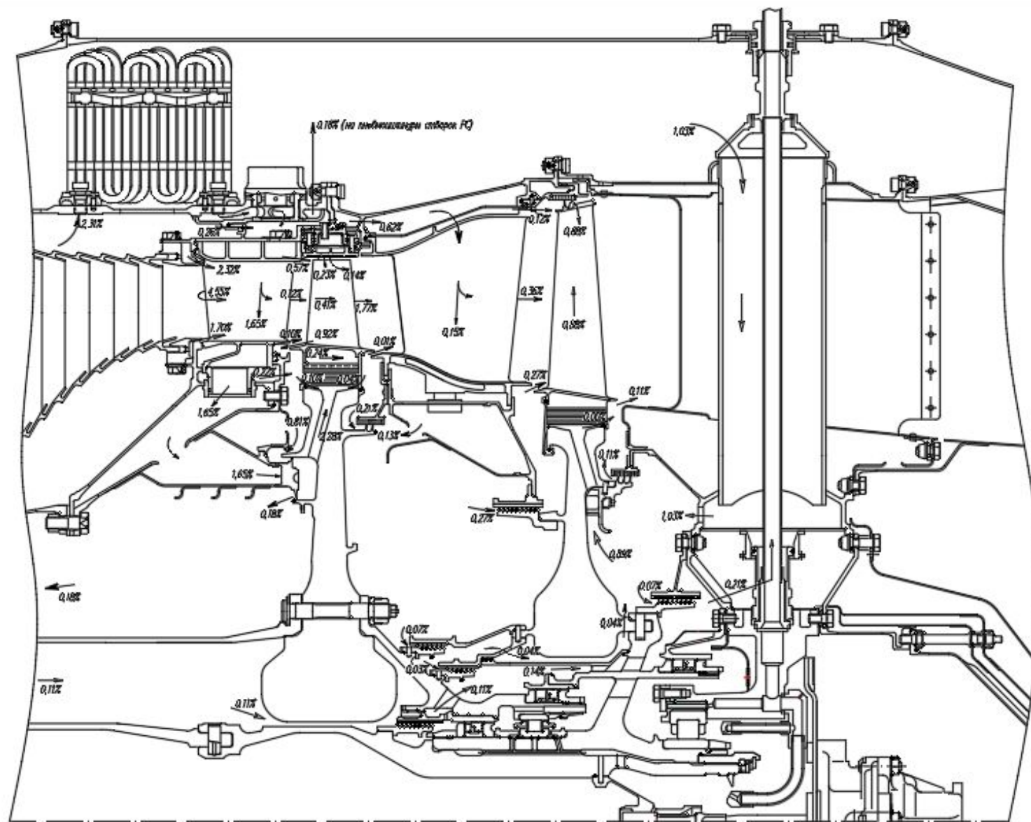
Рисунок 2. Схема охлаждения турбины изд. "99M2". Частичное охлаждение.
