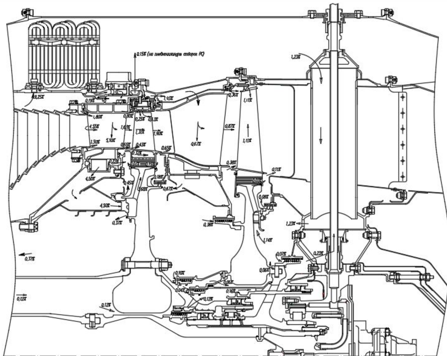
Рисунок 1. Схема охлаждения турбины изд. "99M2". Полное охлаждение.
