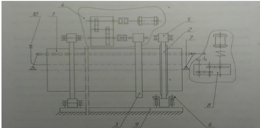
Рис. 1.3. Кінематична схема барабанного змішувача–огрудковувача: 1 – барабан; 2 – бандаж; 3 – зубчатий вінець; 4 – привод обертання барабана; 5 – опорні ролики; 6 – упорні ролики; 7 – очисний пристрій; 8 – привод очисного пристрою; 9 – рама; 10 – установка для зволоження шихти
