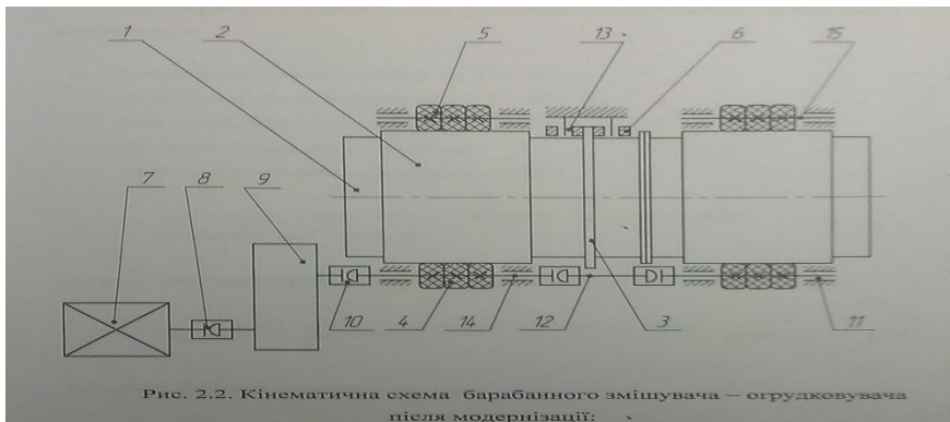
Рис. 2.2. Кінематична схема барабанного змішувача – огрудковувача після модернізації: 1 – барабан; 2 – бандаж опорний; 3 – бандаж упорний; 4 – ролик гумірований опорний приводний; 5 – ролик гумірований опорний холостий; 6 – ролик упорний; 7 – електродвигун; 8 – муфта швидкохідна; 9 – редуктор; 10 – муфта швидкохідна; 11 – підшипник ролика опорного; 12 – промвал; 13 – підшипник ролика упорного; 14 – вал ролика опорного приводного; 15 – вісь ролика упорного.
