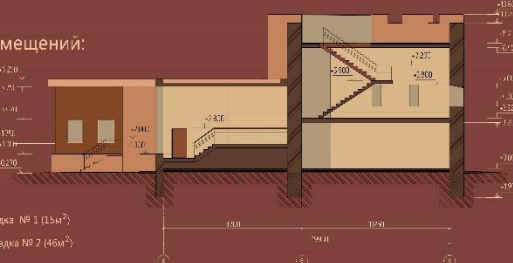
Разрез 1 - 1, М 1:100
