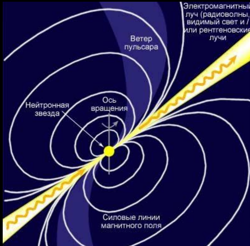
Модель пульсара
