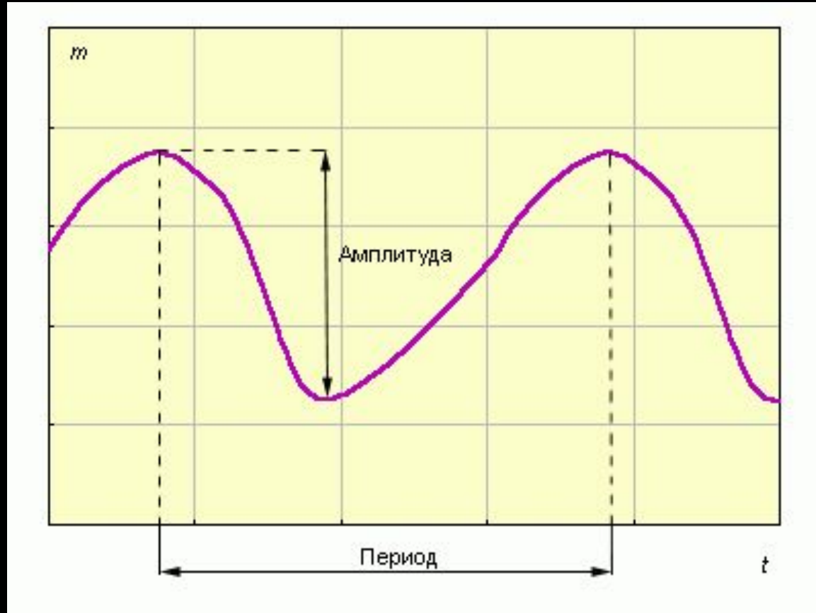
Амплитуда и период переменной звезды
