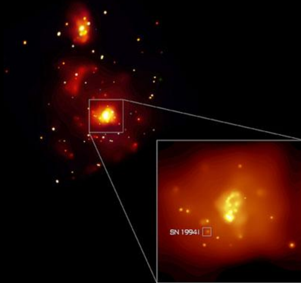
Рентгеновское излучение на месте вспышки SN 1994I
