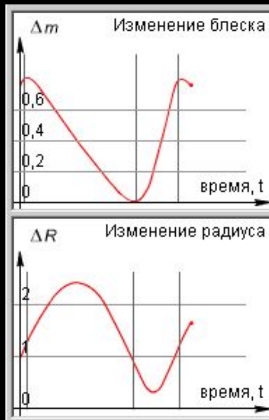
Цефеиды
