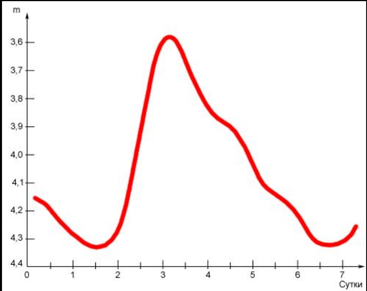
Кривая блеска звезды Дельта Цефея
