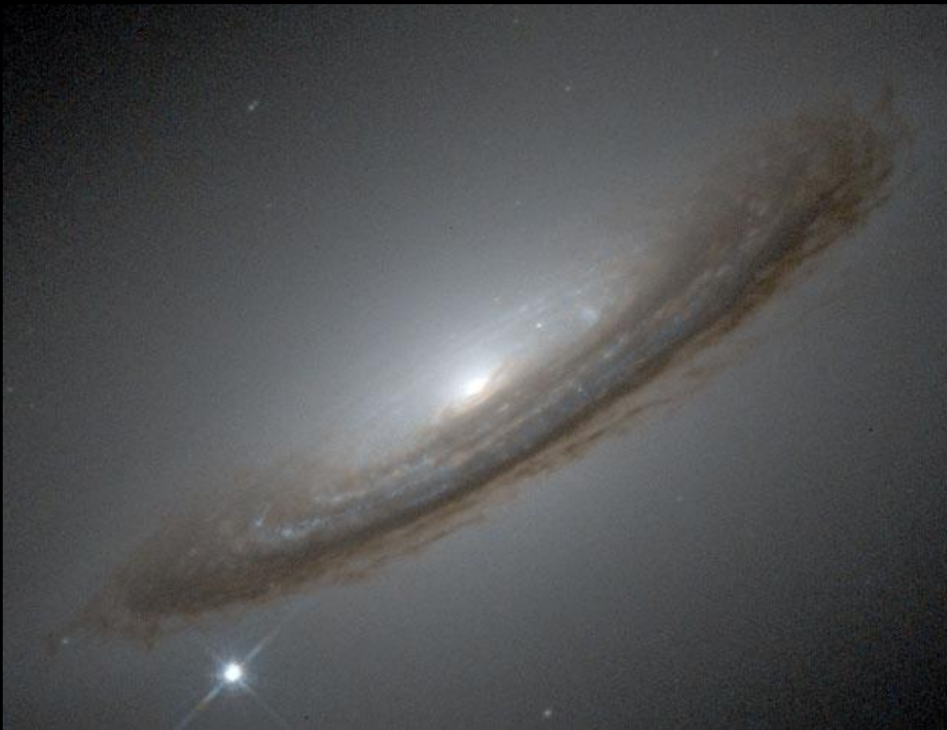
Сверхновая звезда 1994 года, вспыхнувшая на краю спиральной галактики
