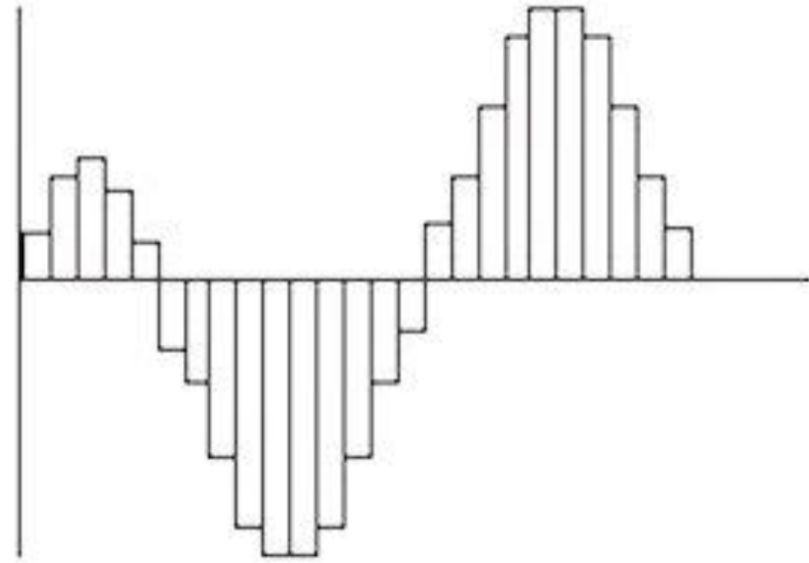
Цифровой звук
