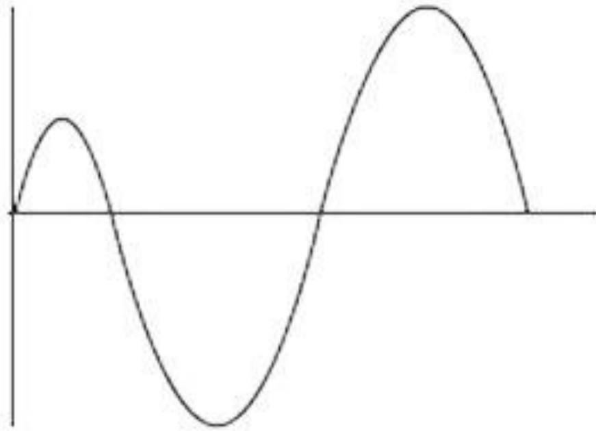
Аналоговый звук
