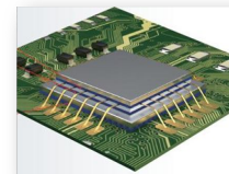
Стек из кристаллов одного размера без смещения и без переходников (DOW Die-on-Wires)
