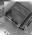
Стек из кристаллов одного размера со смещением
