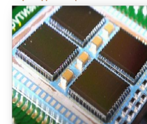
Стек с сочетанием проволочного и flip-chip монтажа кристаллов
