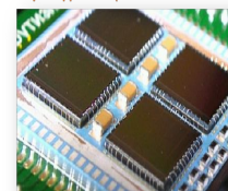
Стек с сочетанием проволочного и flip-chip монтажа кристаллов
