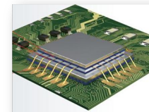
Стек из кристаллов одного размера без смещения и без переходников (DOW Die-on-Wires)
