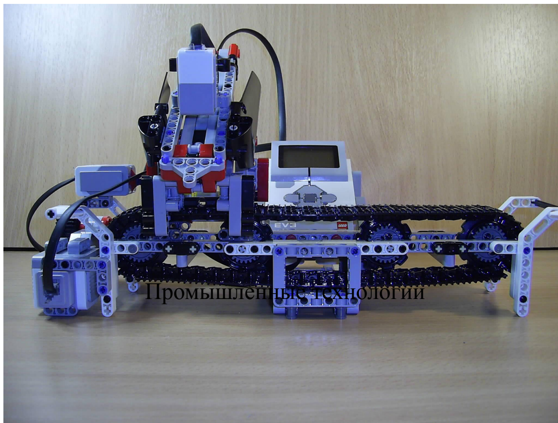
Прототип робота-сортировщика на базе конструктора Lego Mindstorms EV3
