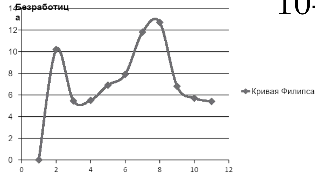
Кривая Филипса
