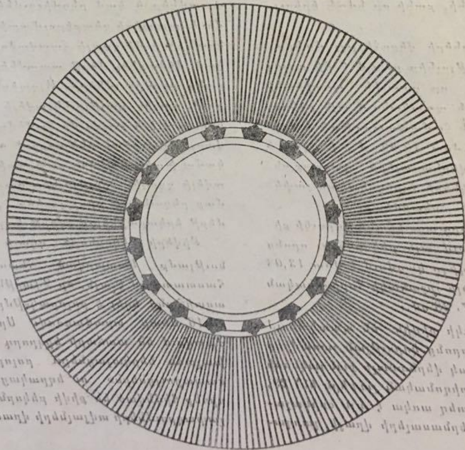
Գծ. 11. Զվարթնոցի երրորդ աստիճանի (գմբեքաքմբուկի) հատակագիծ
