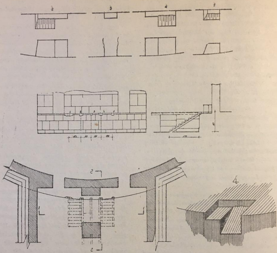
Գծ. 6. Ներհանարյ իշնոյ սանդուխտներ ճեմապատի եզրաշերտի վրա— շափագրություն
