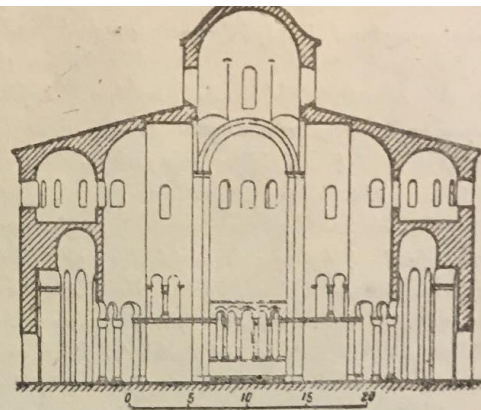
Ժ. 20. Քանա տանարի կտրվածք
