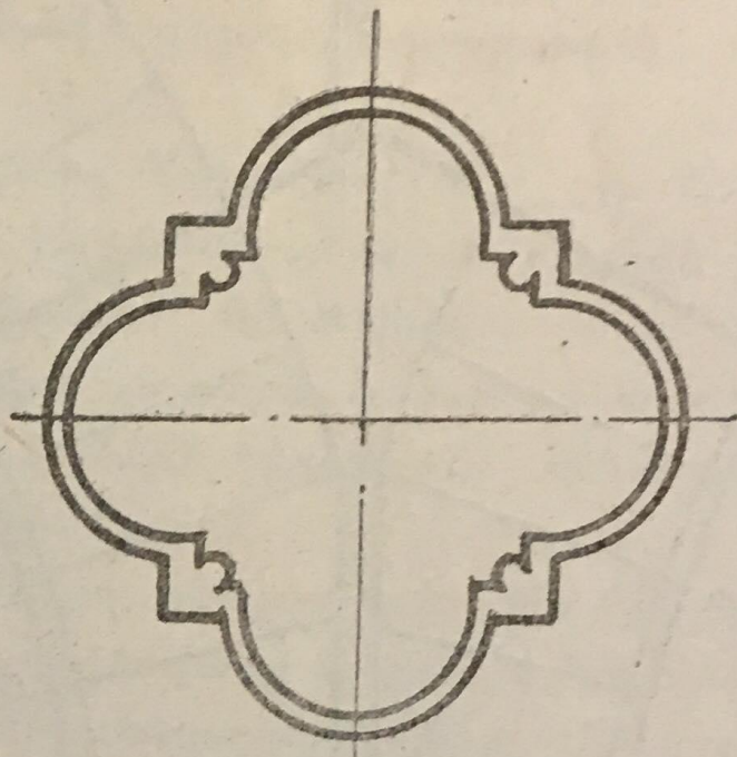
Պժ. 9. Տանարի երկրորդ աստիճանի հատակագծի պարագիծը ըստ Կուզնեցովի (1951 թ.) և ըստ Մնացականյանի (1959 թ.)
