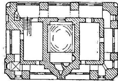
План 1—1
