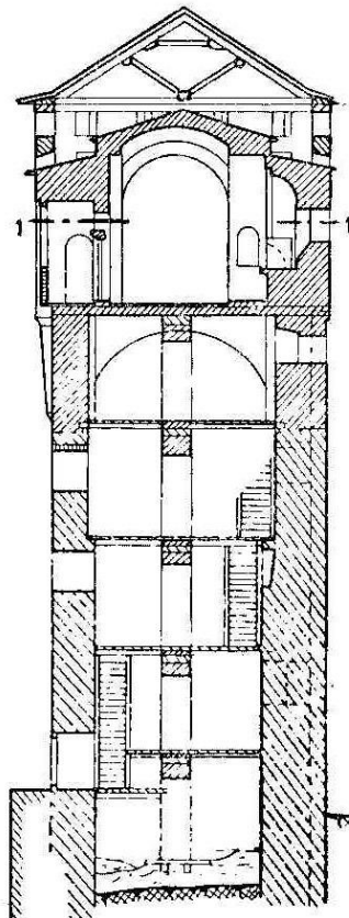
Поперечный разрез
