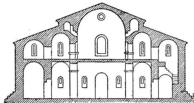
Поперечный разрез
