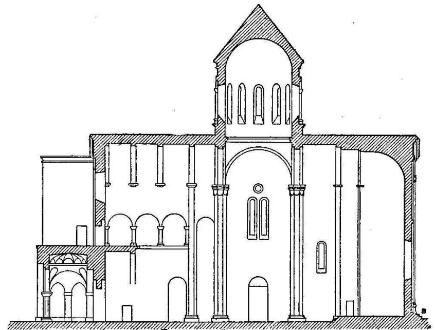
Продольный разрез
