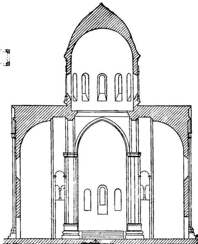
Поперечный разрез
