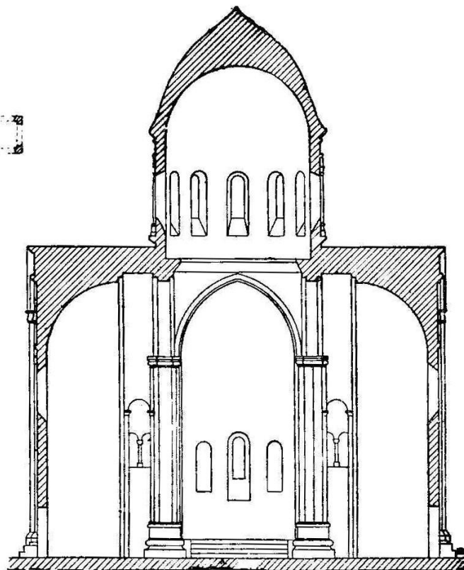
Поперечный разрез
