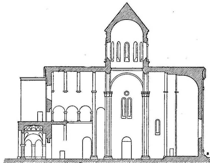
Продольный разрез
