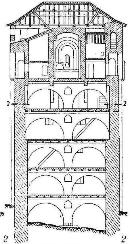
Продольный разрез
