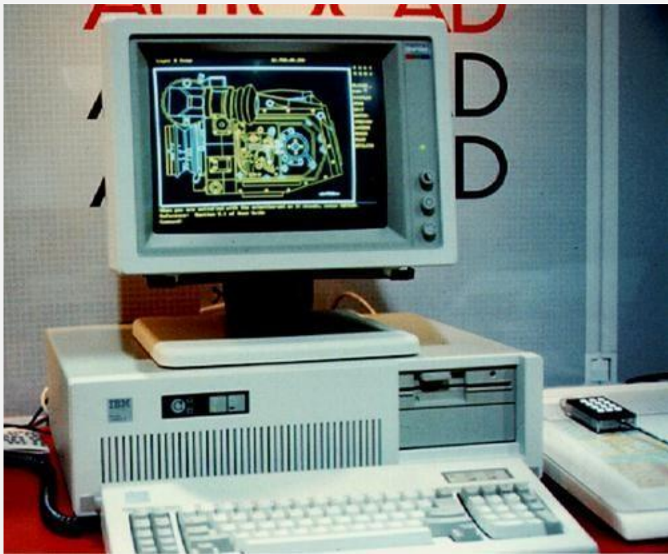
1982: AutoCAD v1.0
