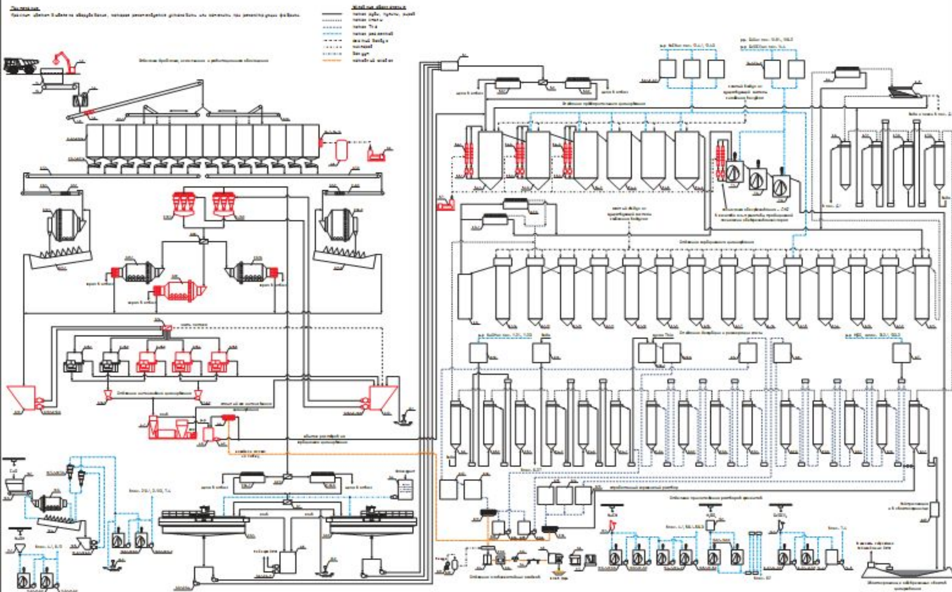
Приложение 3 Схема цепи аппаратов обогатительной фабрики по переработке руды месторождения «Многовершинное» (после реконструкции).
