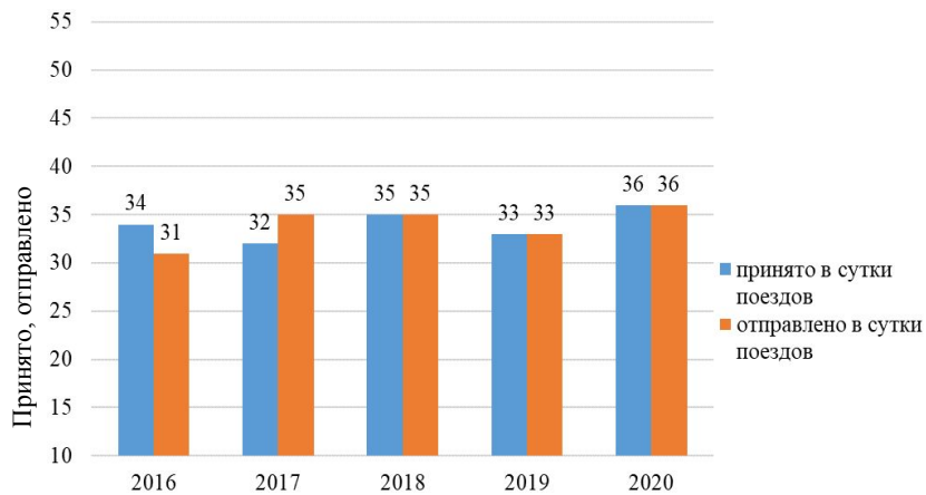
Рисунок 2.3 – Суточный прием и отправление поездов в 2016-2020 годах по станции Витебск
