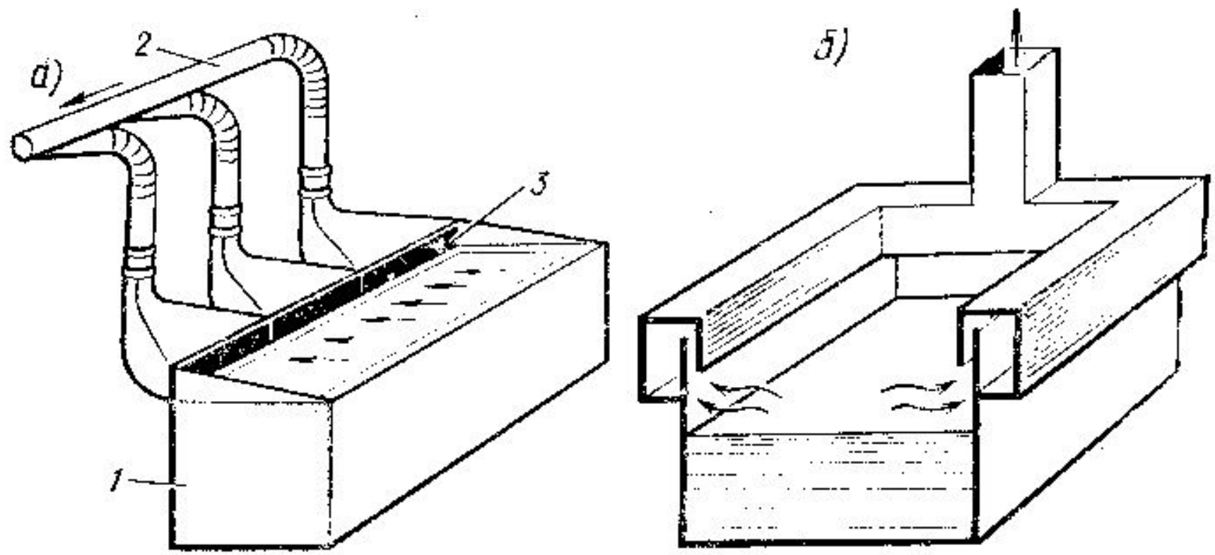
Рис. 19 Бортивые вытяжные устройства
