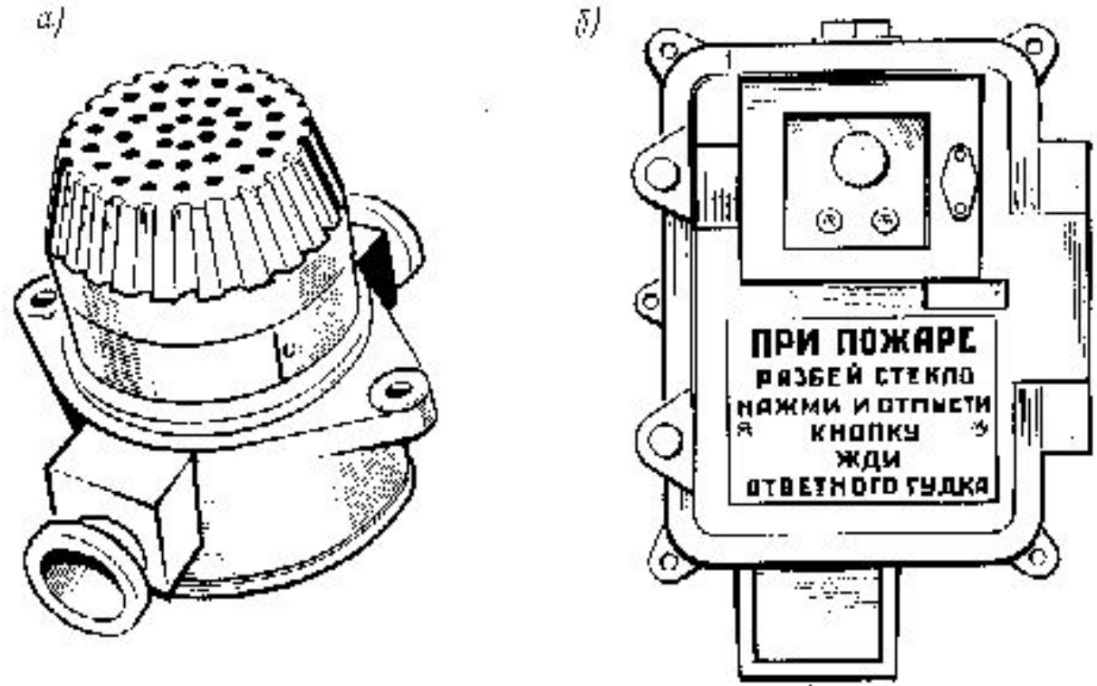
Рис. 49 Пожарные извещатели: а - автоматический; б - ручной.
