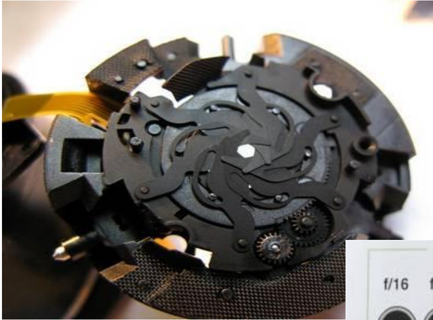
Шестилепестковая диафрагма
