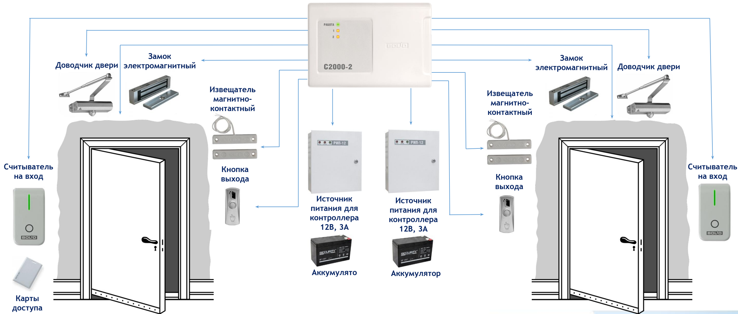
C2000-2 Контроллер доступа
