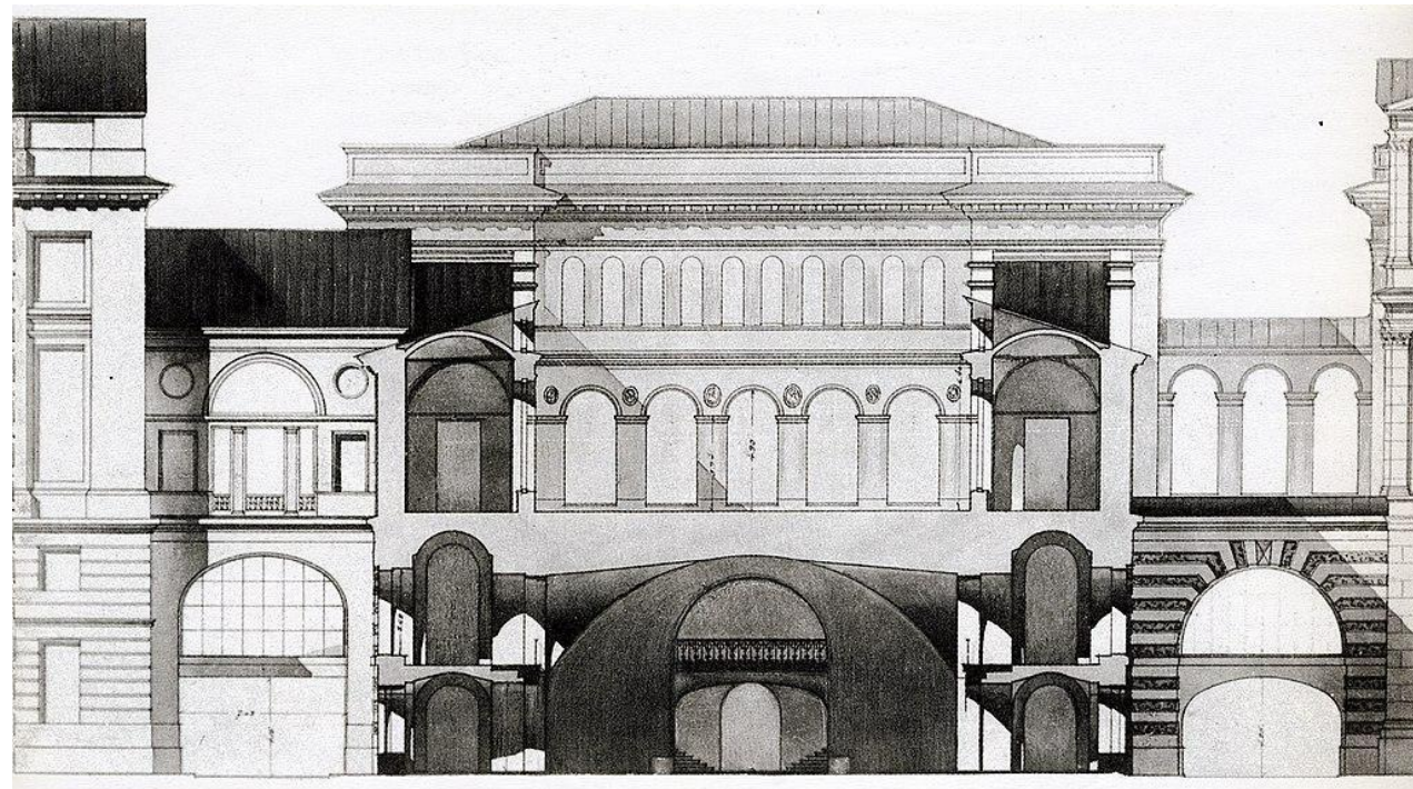
Поперечный разрез
