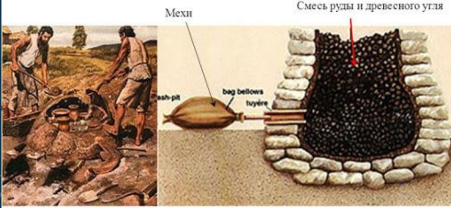
Схема давньої печі
