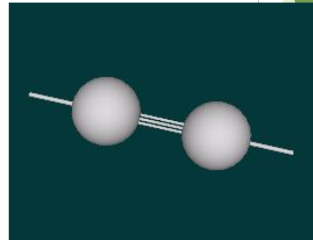
Тройная связь
