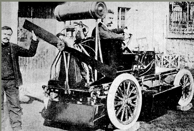
Опытная машина Siders конструкции Гарбаччо. 1913 год
