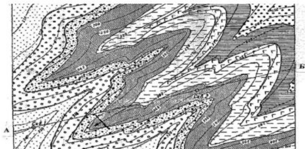
Структурная геология
