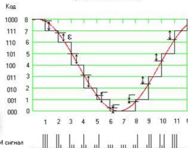
Преобразование непрерывного сообщения в трехзначный ИКМ сигнал
