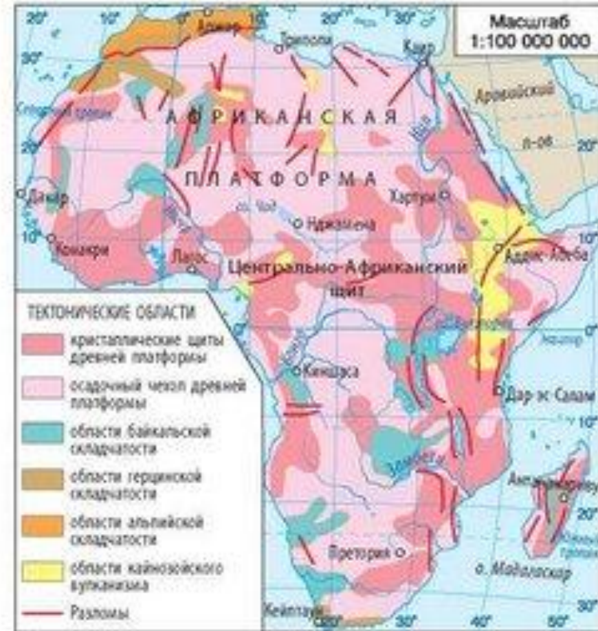
Рис. 1. Тектоническое строение Африки.
