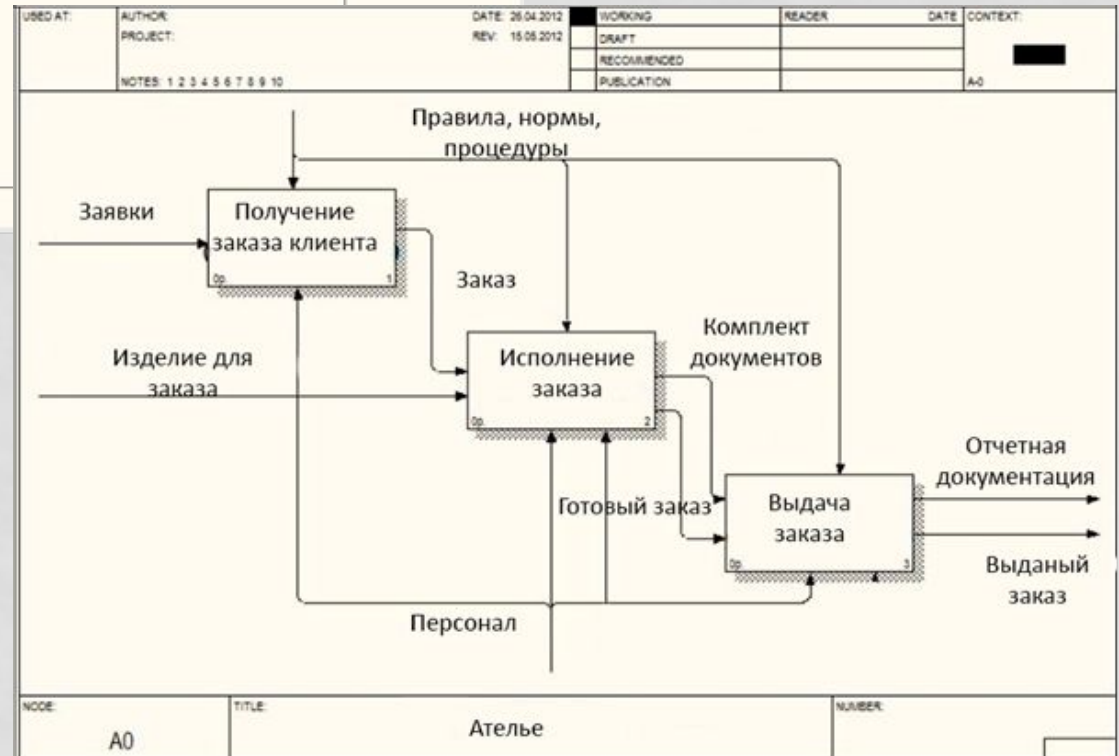
Модель бизнес-процессов верхнего уровня в нотации IDEF0 (декомпозиция концептуальной схемы)
