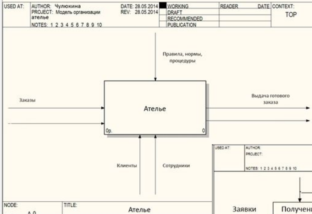
Контекстная диаграмма компании «Заплата» в нотации IDEF0
