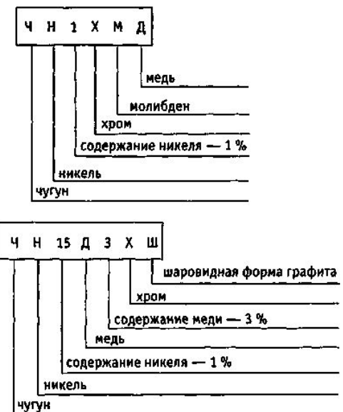
Пример маркировки коррозионно-стойкого чугуна
